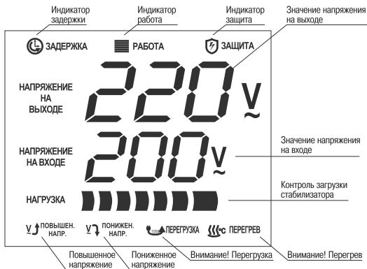
Рис 2. Индикация режимов работы настенных стабилизаторов
