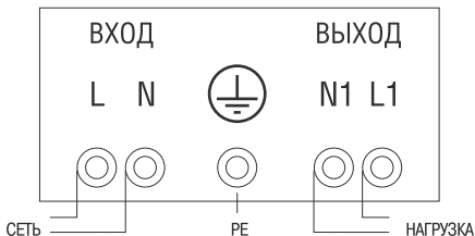
Рис 4. Схема подключения стабилизаторов
